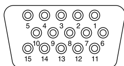
D-SUB
